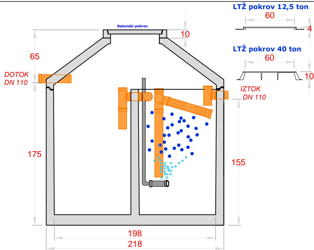
Možnost postavitve iztoka v desno stran
